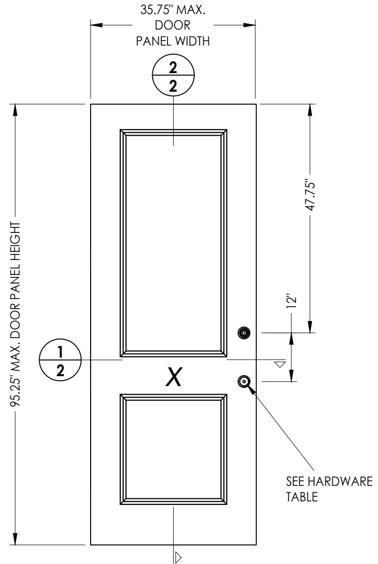
40 DOOR PANEL
